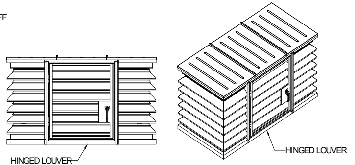
HINGED DOOR
